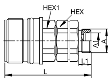
24° 锥外螺纹
