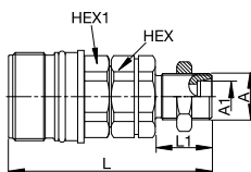
24° 锥外螺纹 - 隔板式
