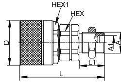
24° 锥外螺纹 - 隔板式
