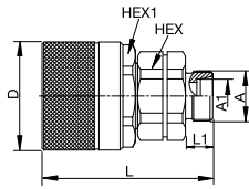
24° 锥外螺纹
